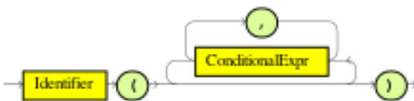
AccumulateInit
