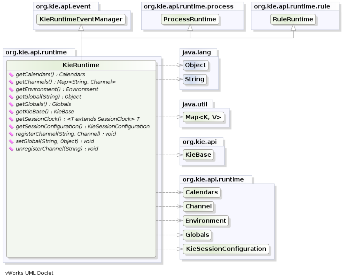
Figure 4.17. KieRuntime
