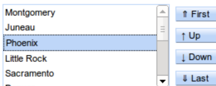
Figure 8.10. <rich:select>
