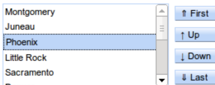
Figure 8.10. <rich:select>
