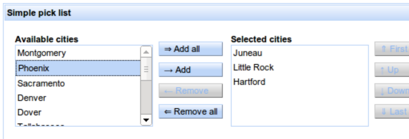
Figure 8.9. &lt;rich:select&gt;
