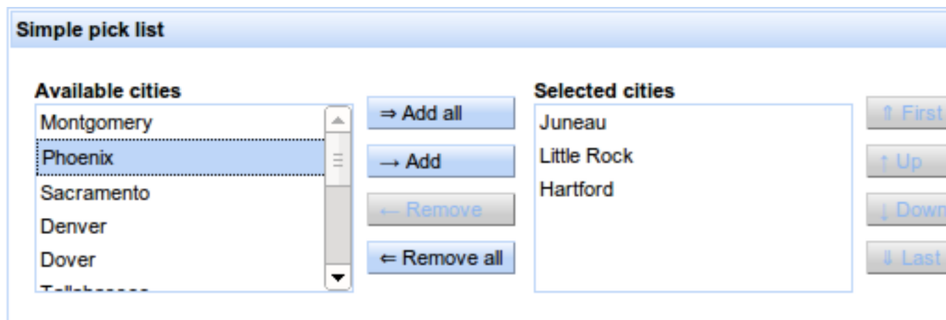
Figure 8.9. &lt;rich:select&gt;
