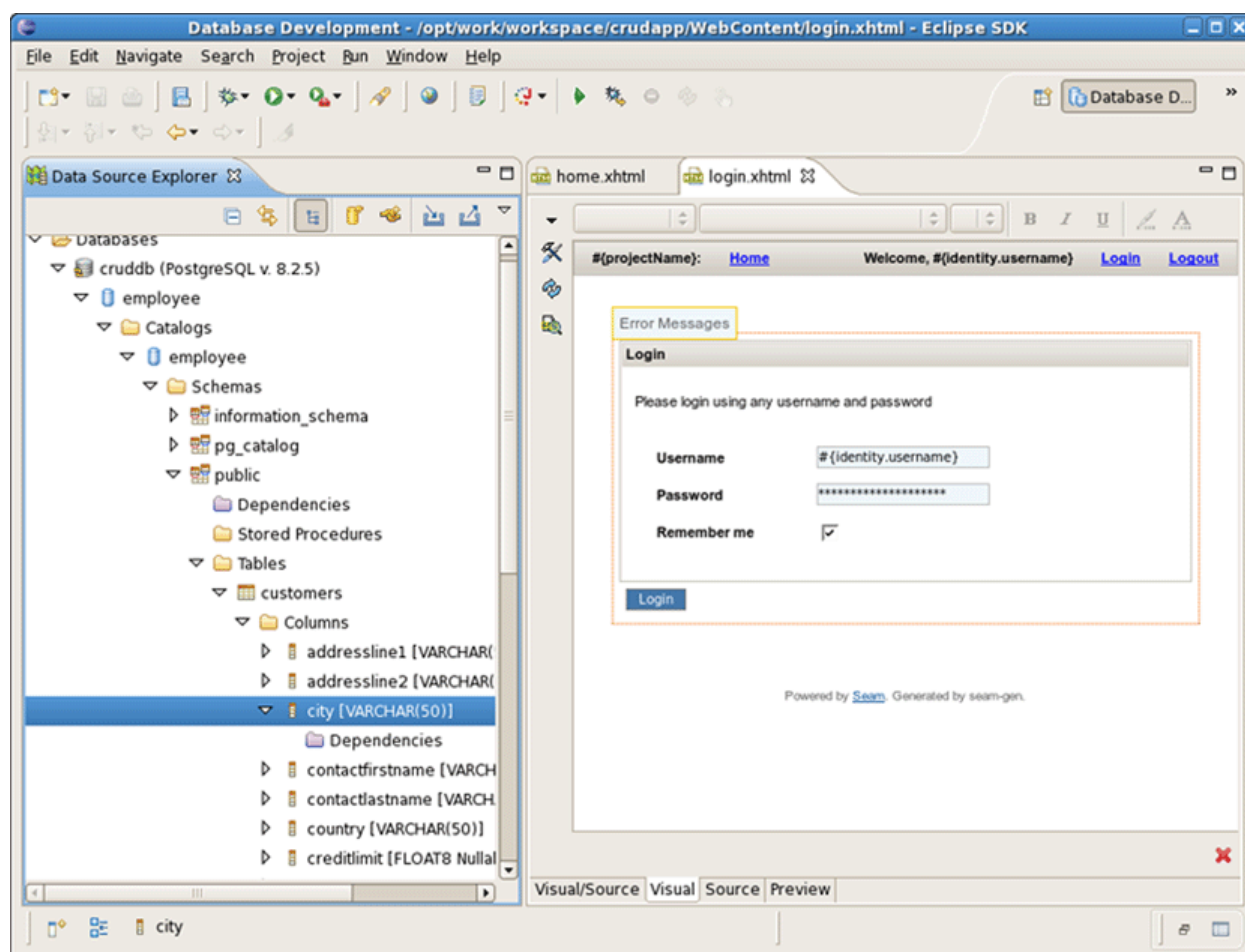
Figure 10.15. CRUDB Database
